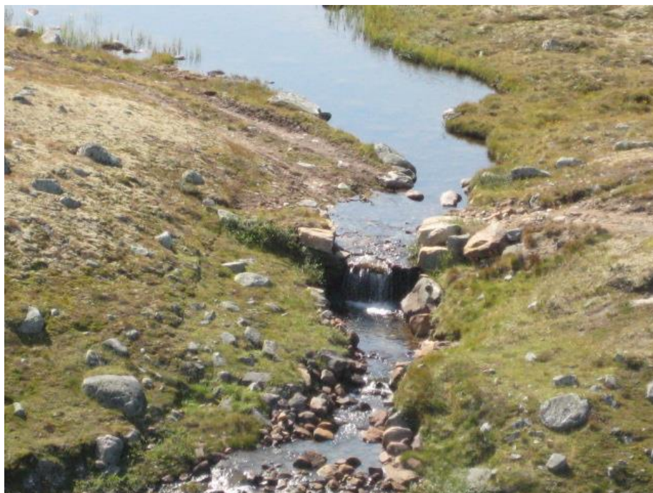
Fig. 12. Ørekytesperre ved Holmetjernan i Nore og Uvdal kommune
